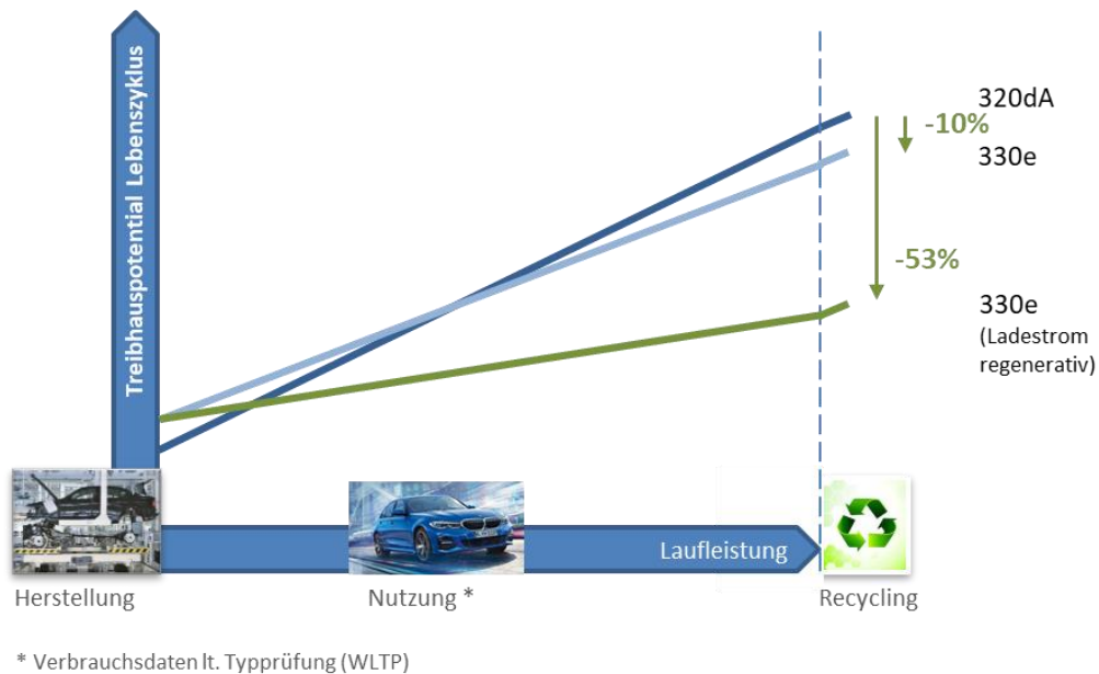
Abb. 3: Einordnung des BMW 330e in Bezug auf ein konventionelles Fahrzeugkonzept (320dA)
