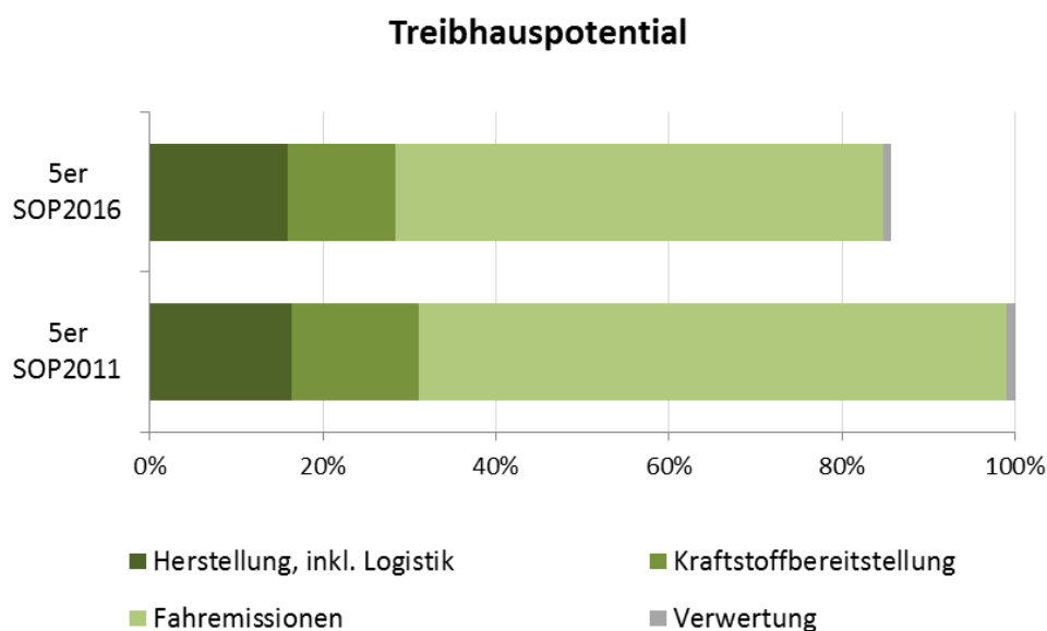
Abb. 2: Verteilung Treibhauspotential über Lebenszyklus des BMW 5er
