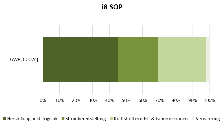
Abb. 2: Verteilung Treibhauspotential über Lebenszyklus des BMW i8
